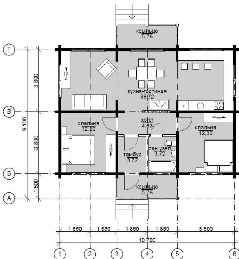
План 1-го этажа
