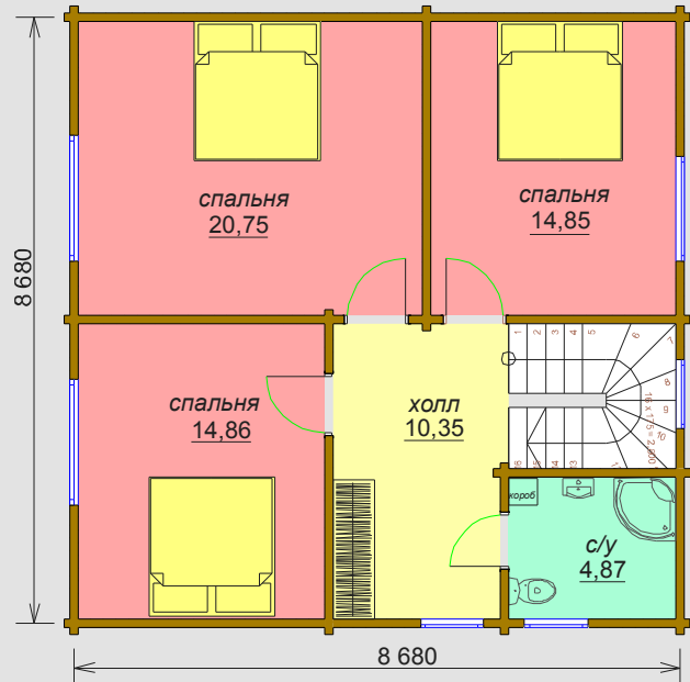
План 2го этажа S= 70,6 м2
