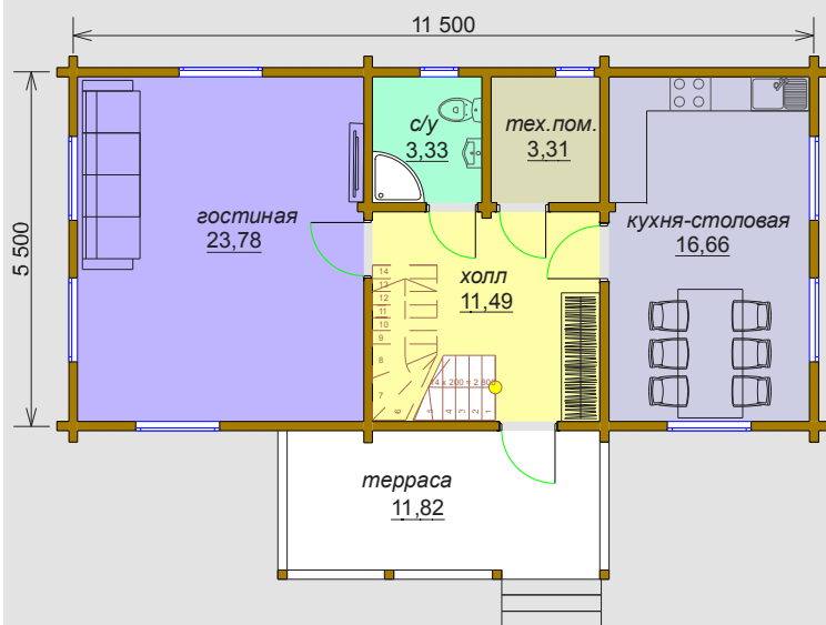
План 1го этажа S= 58,6 м2 (без террасы)
