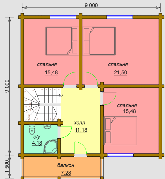
План 2-го этажа S= 75,1
