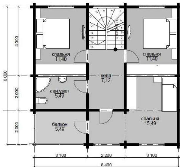
План 2 го
