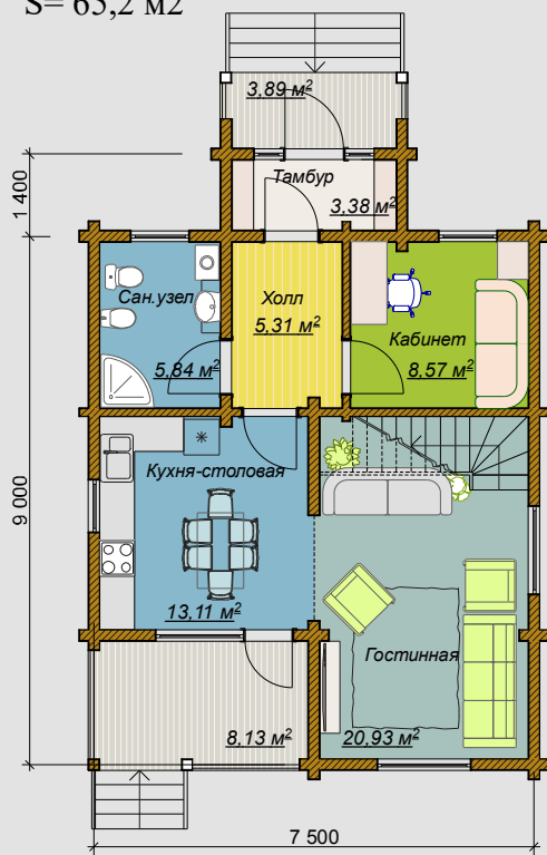
План 1 го этажа S= 65,2 м 2
