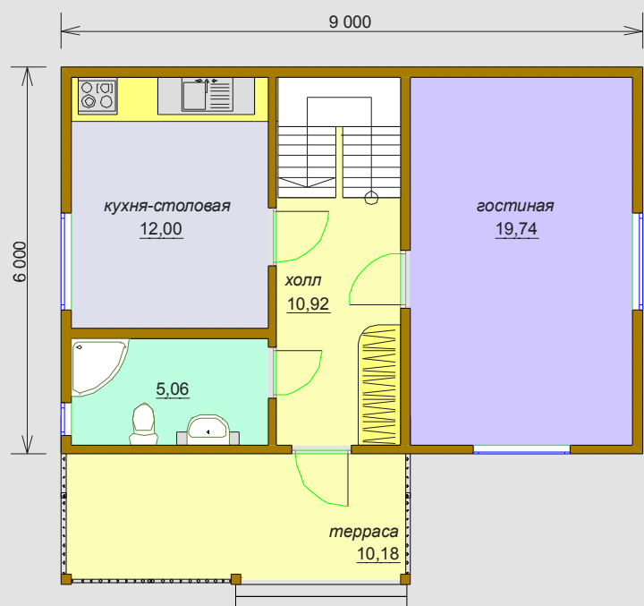
План 1го этажа S= 47,72 м2 (без террасы)
