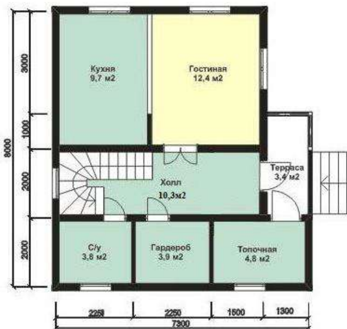
План 1го этажа S= 44,9 м 2 (без крыльца)
