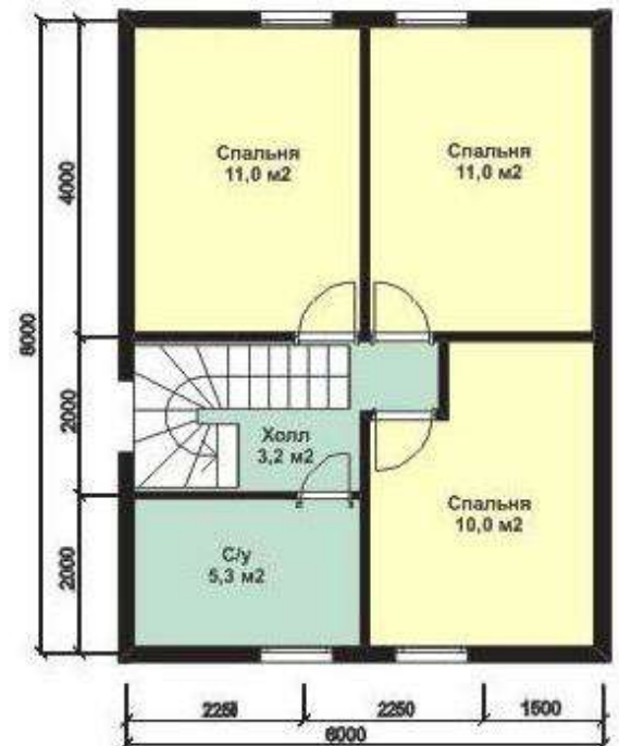
План 2го этажа S= 40,5 м 2
